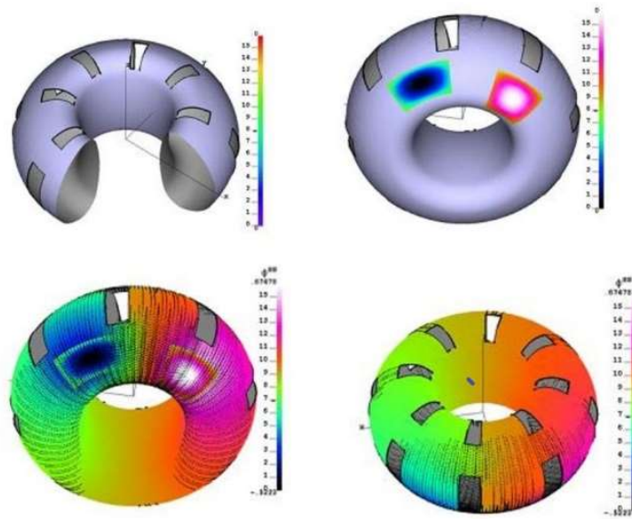
Figura 1. Stanga sus: perete toroidal cu gauri de acces. Dreapta sus: zonele in perete unde este distribuit curentul plasma-perete (scenariu teoretic). Stanga jos: vedere de jos a distributiei potentialului scalar al curentului de divergenta potential nenula. Dreapta jos: Vedere de sus a acelorasi curenti, in mod evident mai mici decat in partea de jos.
